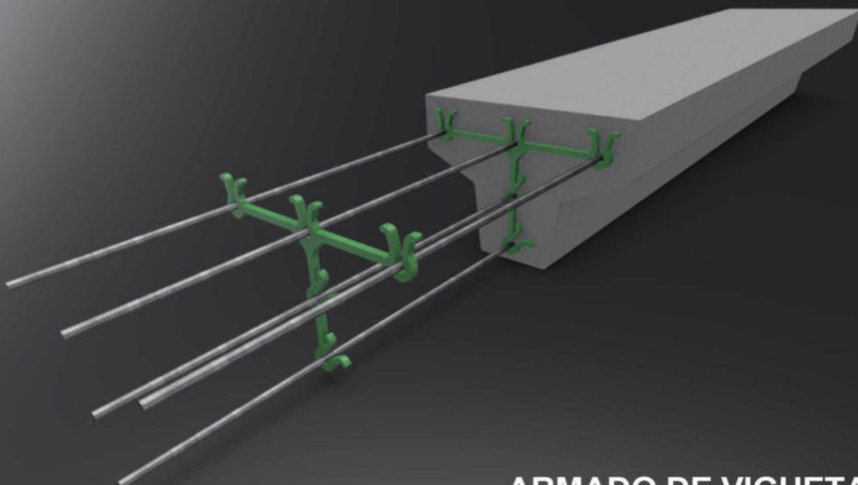
ARMADO DE VIGUETA
